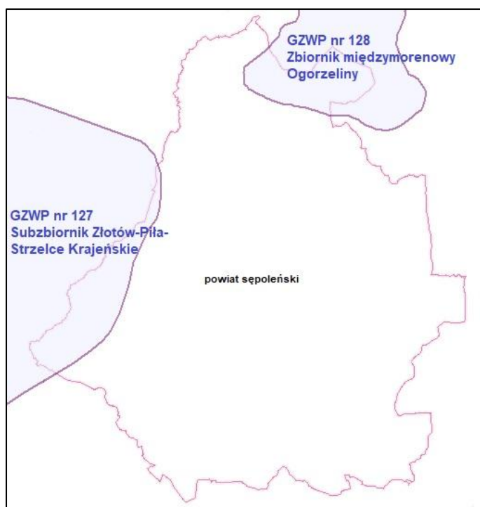
Rysunek 4 Główne Zbiorniki Wód Podziemnych (GZWP) oraz jednolite części wód podziemnych (JCWPd) na terenie powiatu sępoleńskiego (źródło: pig.gov.pl)
