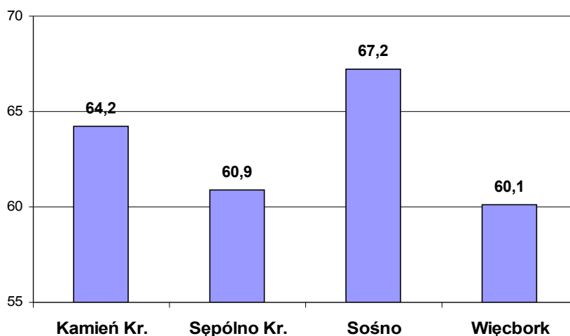
Wskaźnik jakości Rolniczej Przestrzeni Produkcyjnej
