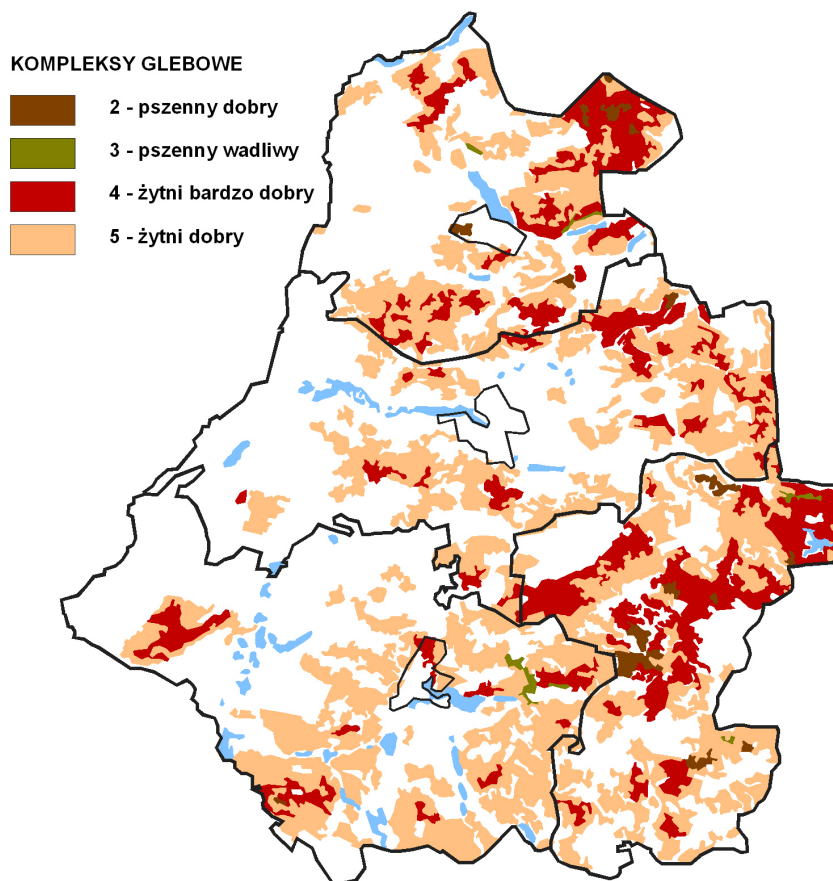
Rys. Rozmieszczenie najlepszych kompleksów glebowych w gminach powiatu (dane GUS 2006 r.)
